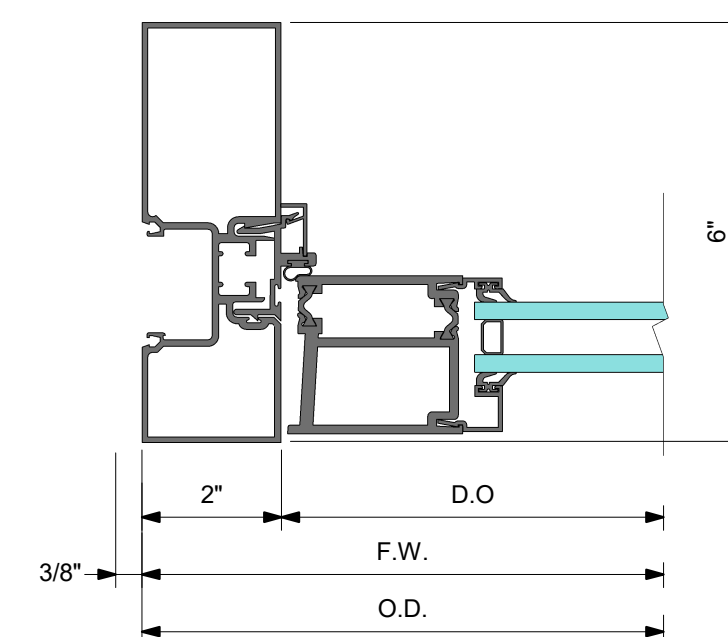
4 DETAIL 4 DOOR JAMB
