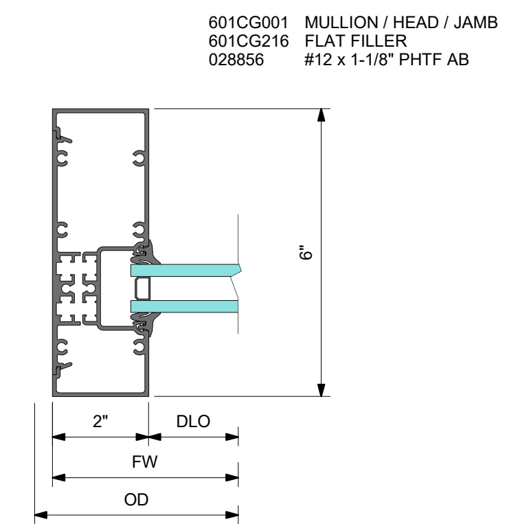
4 DETAIL 4 JAMB
