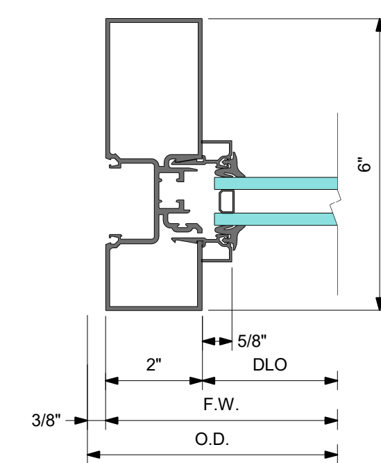
4A DETAIL 4A TRANSOM JAMB
