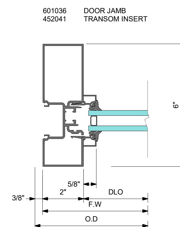
4A DETAIL 4A TRANSOM JAMB
