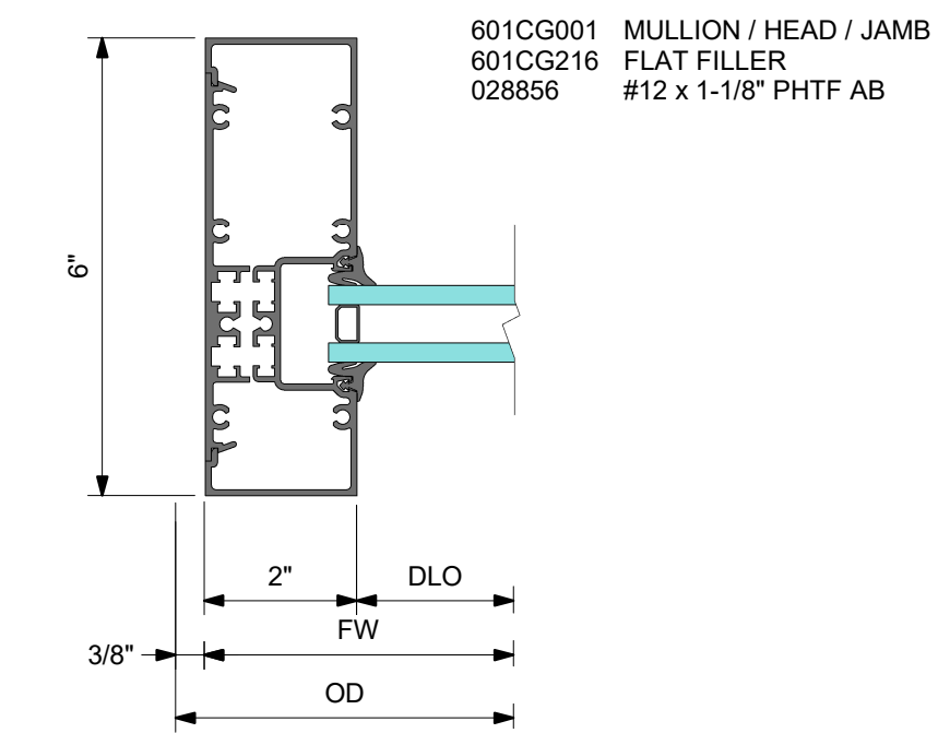
4 DETAIL 4 JAMB
