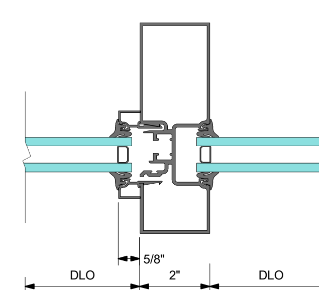
601036 DOOR JAMB 452041 TRANSOM INSERT
